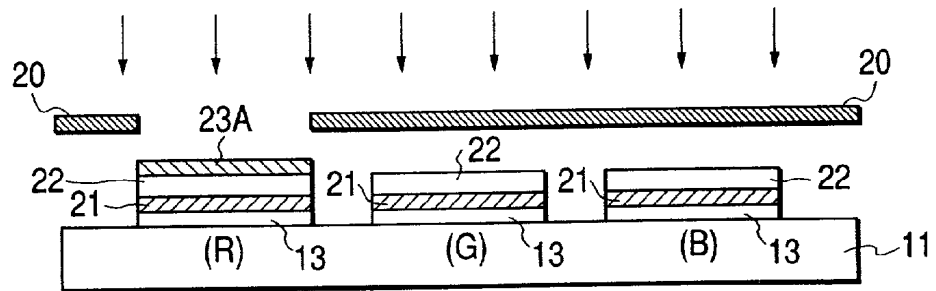
FIG. 11A
